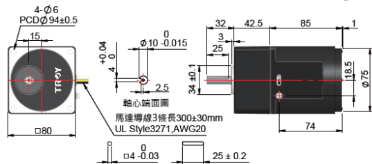
齒輪軸機型 8R25P-□N+8AN□
