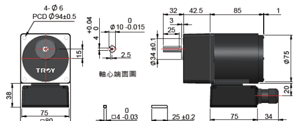
齒輪軸機型 8I25PB-□N+8AN□
