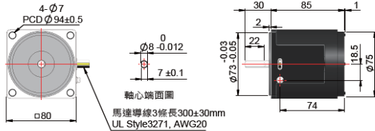
圓軸機型 8I25S-□N
