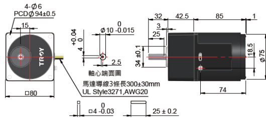
齒輪軸機型 8I25P-□N+8AN□
