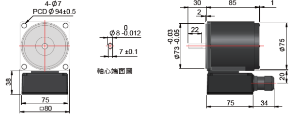
齒輪軸機型 8I25PB-□N+8AN□
