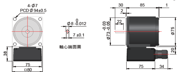
齒輪軸機型 8R25PB-□N+8AN□
