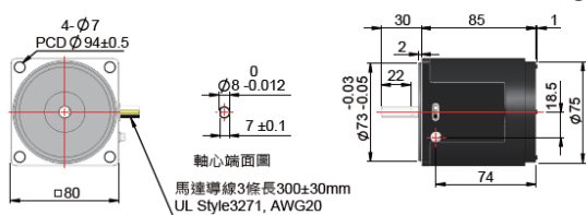
圓軸機型 8R25S-□N
